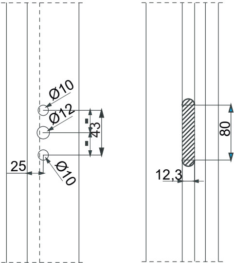
DESENHO DE USINAGEM NO PERFIL
