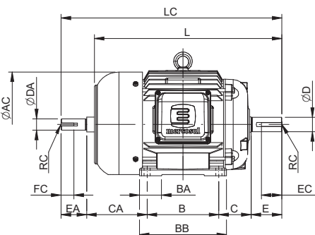
VISTA DO MOTOR COM TAMPA TRASEIRA NORMAL
