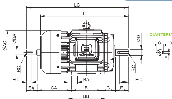
VISTA DO MOTOR COM TAMPA TRASEIRA ALTA EXEMPLO: L100L
