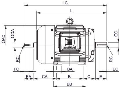
VISTA DO MOTOR COM TAMPA TRASEIRA NORMAL
