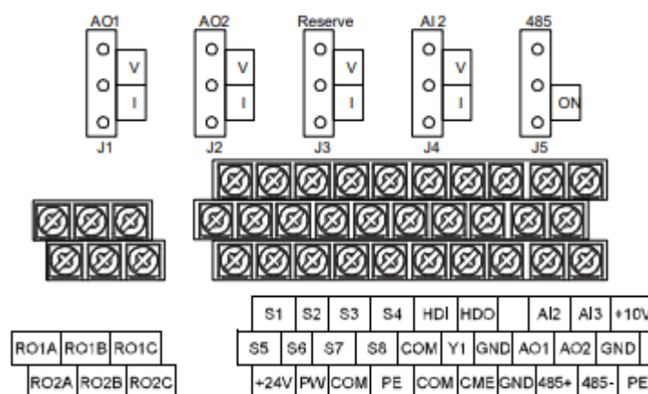
Figura 1 - Para modelos 15kW/18kW(20/25CV) e menores.
