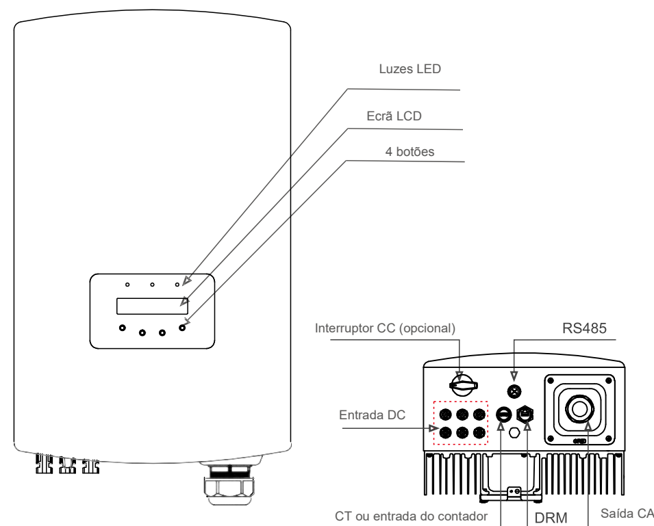
▲ Figura 1.1 Vista frontal
