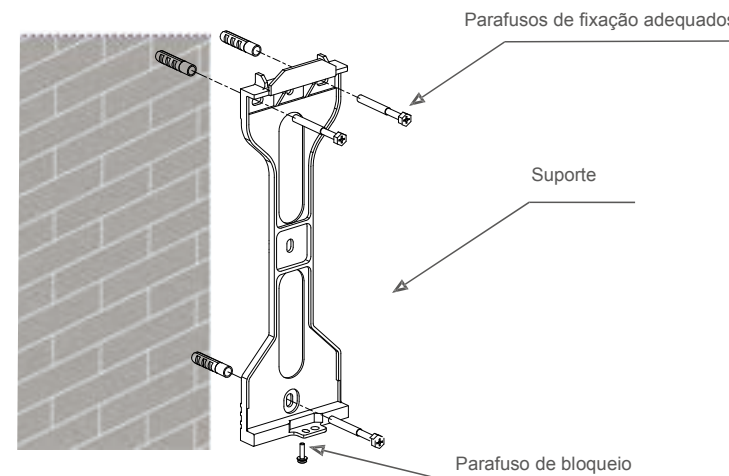
▲ Figura 4.4 Montagem do inversor na parede
