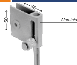
Cód.: 1800 Trinco para janela de correr frontal
