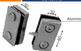
Cód.: 1710 M Mini conjunto mão de amigo para portas de correr
