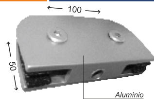
Cód.: 1231 Dobradiça para basculante 50x100mm
