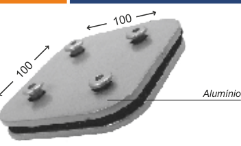
Cód.: 1316 Suporte sem núcleo para união de 4 vidros
