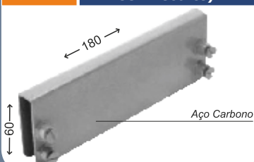
Cód.: 1906 P Suporte para mola aérea (Porta - sem recorte)
