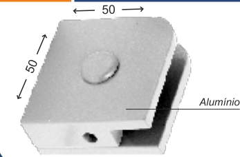
Cód.: 1308 Suporte para união de 3 vidros (com núcleo)
