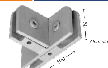
Cód.: 1308 Suporte para união de 3 vidros (com núcleo)
