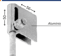
Cód.: 1800 S Trinco de pressão para janela de correr frontal
