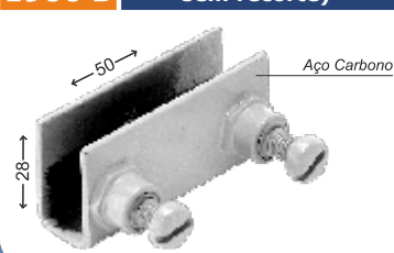
Cód.: 1906 B Suporte para mola aérea (Bandeira - sem recorte)
