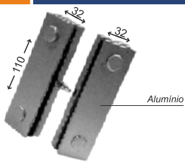
Cód.: 1710 Conjunto mão de amigo para portas de correr
