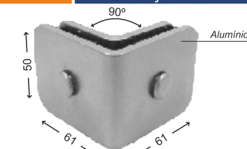
Cód.: 1320 Suporte central para união de 2 vidros instalação a 90°
