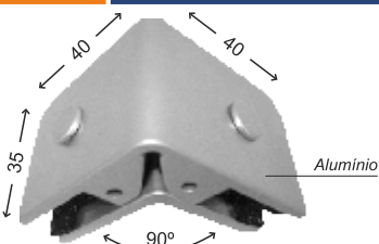
Cód.: 1321 Suporte piso/teto para união de 2 vidros a 90°
