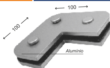
Cód.: 1310 Suporte sem núcleo para união de 3 vidros
