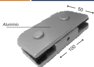
Cód.: 1306 Suporte para união de 2 vidros
