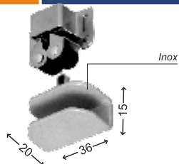
Cód.: 1704 Fecho de pressão para portas de extintores
