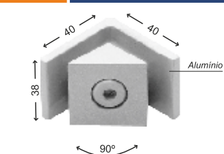
Cód.: 1322 Suporte de centro para união de 2 vidros a 90°
