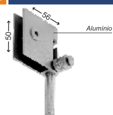
Cód.: 1810 D Trinco direito para janela de correr
