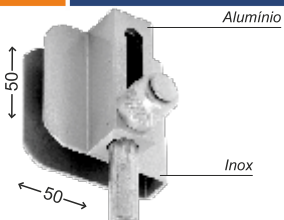
Cód.: 1800 B Trinco de pressão lateral para janela de correr
