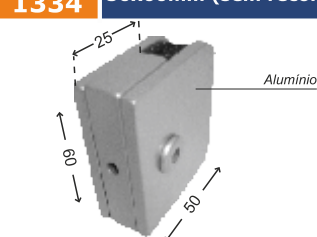
Cód.: 1334 Grapa para sacadas 50x60mm (sem recorte)
