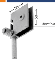
Cód.: 1810 E Trinco esquerdo para janela de correr
