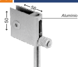
Cód.: 1800 A Trinco para janela de correr lateral
