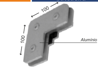
Cód.: 1315 Suporte sem núcleo para união de 3 vidros com batedeira
