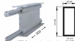
CHU 072-3 Chumbador Lm008 alumínio 300mm
