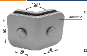
Cód.: 1322 A Suporte para união de 2 vidros a 135°
