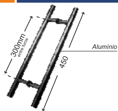
Cód.: 1679 Puxador tubular em "H"
