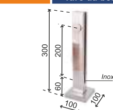
Cód.: 1334 I Grapa 300mm 01 furo 50mm afastamento 200mm furo da borda em Inox
