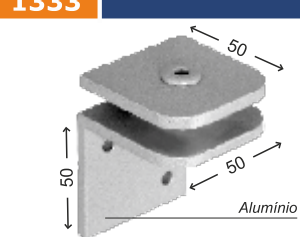
Cód.: 1333 Suporte para prateleiras
