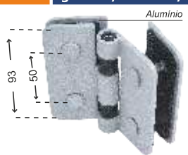
Cód.: 1756 D Dobradiça dupla direita automática granito/madeira/vidro
