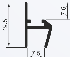
BX-130 0,800 Kg/BARRA 6m
