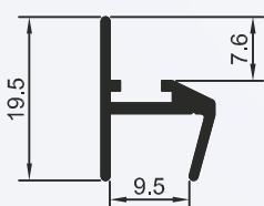
BX-131 0,900 Kg/BARRA 6m
