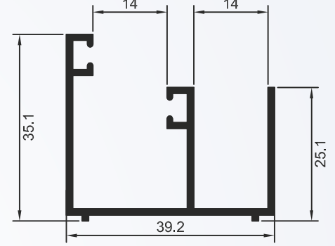
BX-141 2,690 Kg/BARRA 6m
