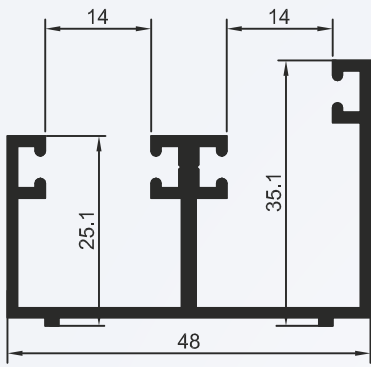
BX-150 3,900 Kg/BARRA 6m
