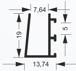
BX-127 0,924 kg/BARRA 6m
