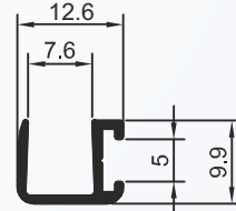
BX-126 0,600 Kg/BARRA 6m
