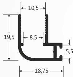
BX-251 1,070 Kg/BARRA 6m
