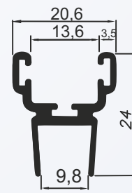
BX-133 1,716 kg/BARRA 6m
